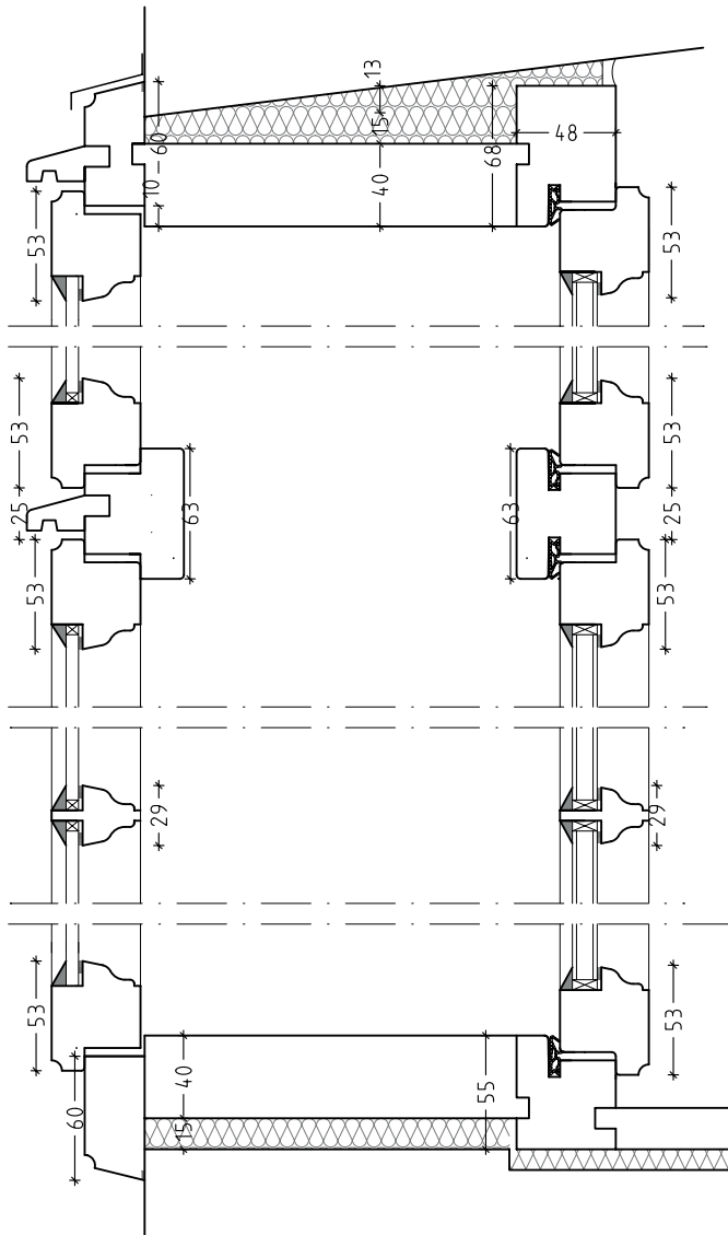
Kastenfenster nach außen aufgehend
