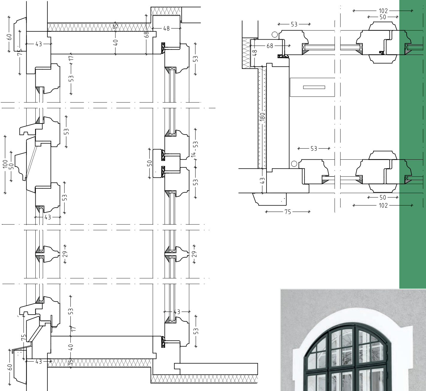
Pfostenstockkastenfenster
