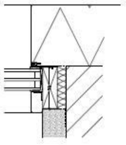
3fach Verglasung
