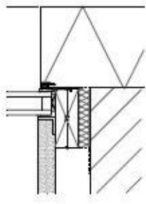
2fach Verglasung
